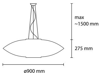
SP UFO 90 3 E27 42W ALO
