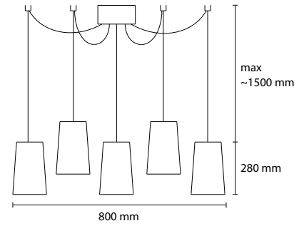
SP PLIZZY 5 / 18 5 E14 28W ALO
