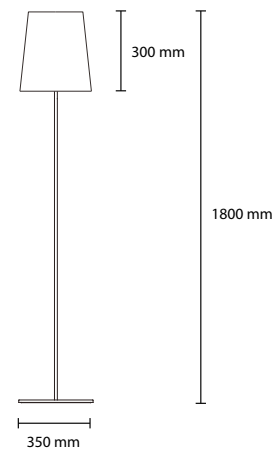
PT PLIZZY 180 1 E27 54W ALO
